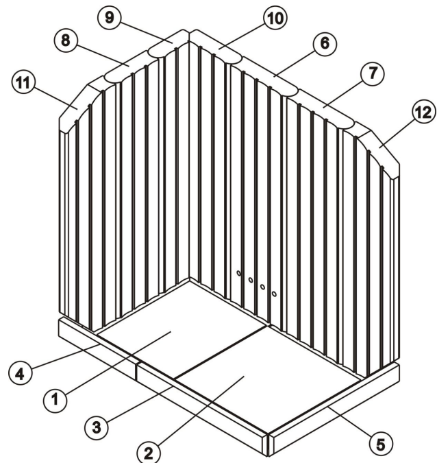
Abb. 1: Zusammenstellung der Schamottesteine Eck-Kamin 57/67/44 STR
